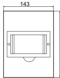
暗盒 6 回路 Flush Mounted MCB Enclosure 6ways
